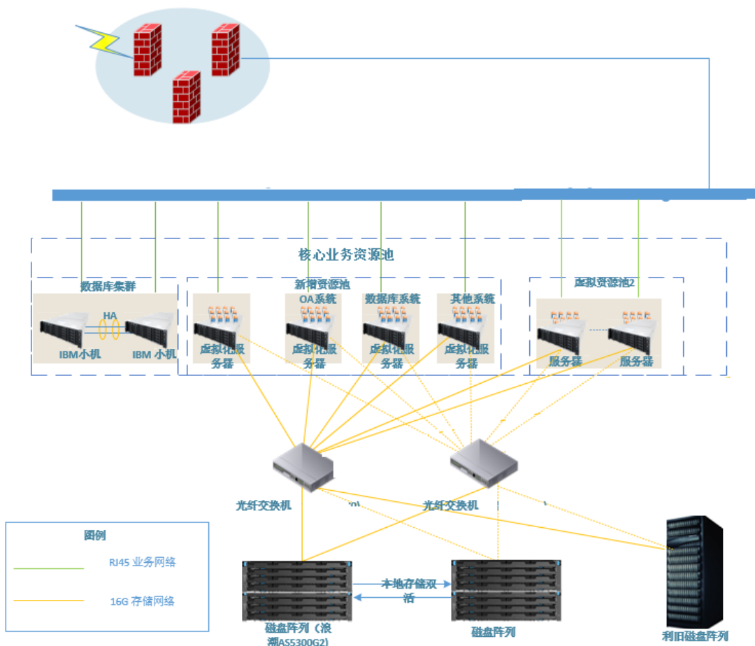
虚拟化平台拓扑图
