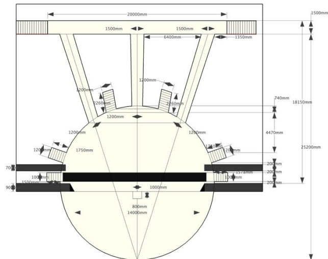
8组功能台阶（6组接圆型平台：建筑台口后2组 假台口后2组 三组通道间2组；2组左右接横向通道）
