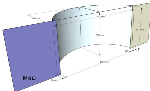
环形幕两侧紧贴假台口内沿。
