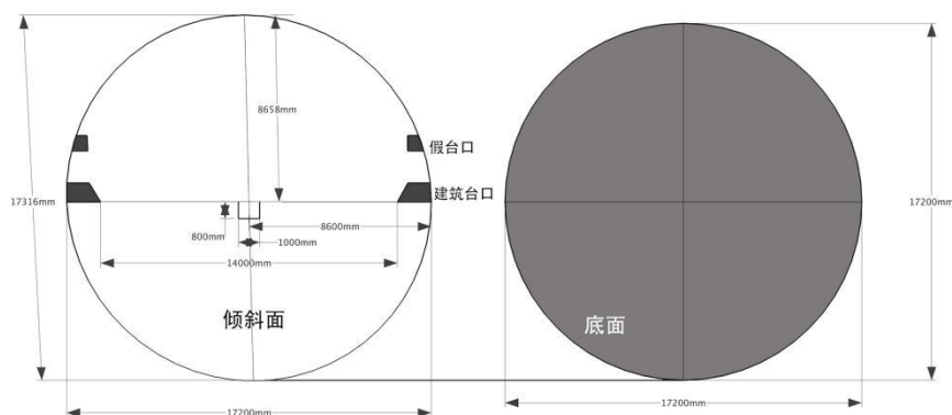
国家大剧院话剧《暴风雨》圆形平台顶视尺寸
