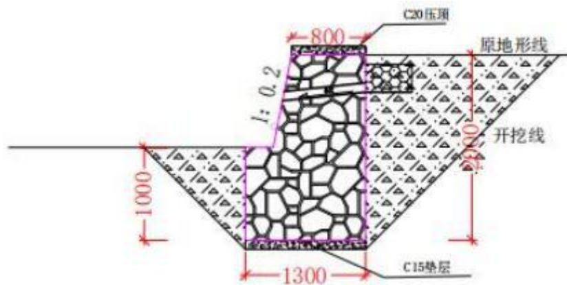
图 3-1DQ01 挡土墙示意图
