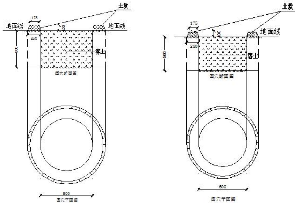
图 2-1A 型树穴大样图图 2-2B 型树穴大样图
